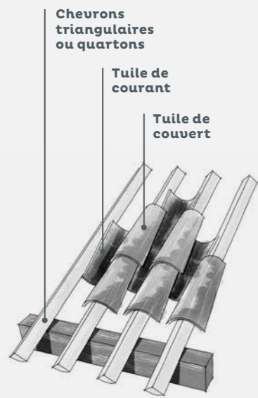
Pose sur chevrons triangulaires ou quarts support discontinu, pose à sec ou scellée
